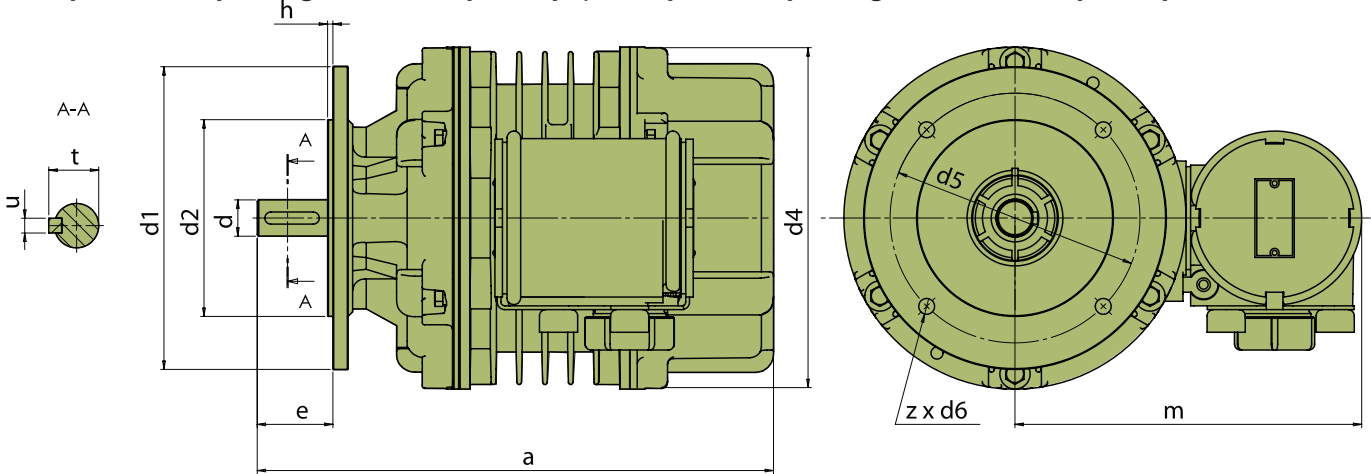
Габаритно – присъединителни размери/ Габаритно-присоединительные размеры
